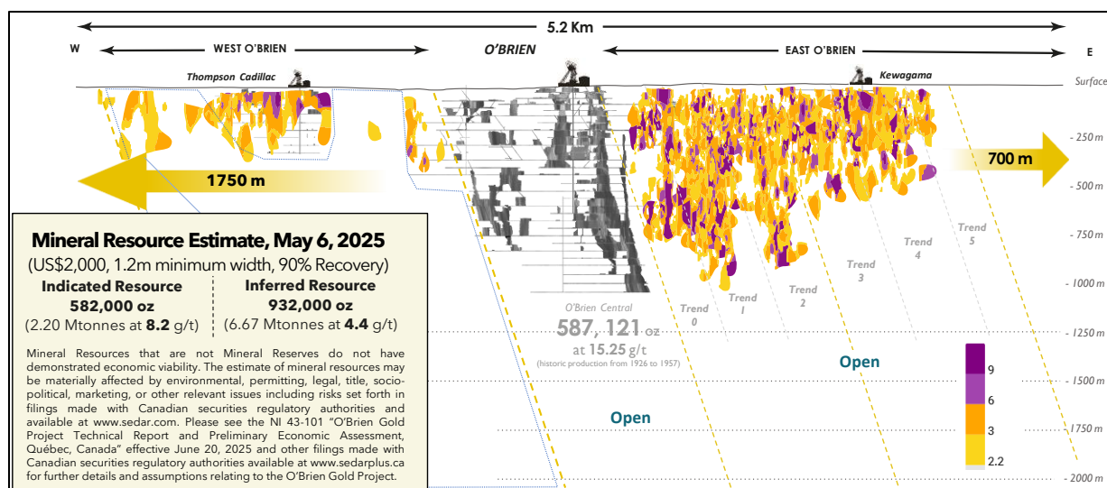
Figure 1 : Le Projet Aurifère O'Brien, de Thompson-Cadillac/O'Brien Ouest, mine O'Brien et jusqu'à O'Brien Est - Vues Longitudinale et en Plan incluant les Ressources Minérales courantes.
