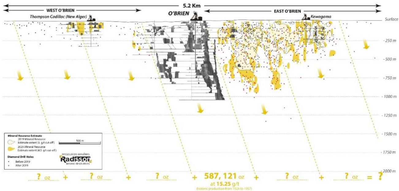
Figure 1. Projet aurifère O'Brien - Vue longitudinale regardant vers le nord – Estimation des ressources minérales 2023 à une teneur de coupure de 4,5 g/t Au
